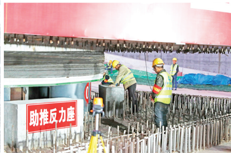
转体过程中,工作人员查看旋转垫盘,掌握转体状况。
